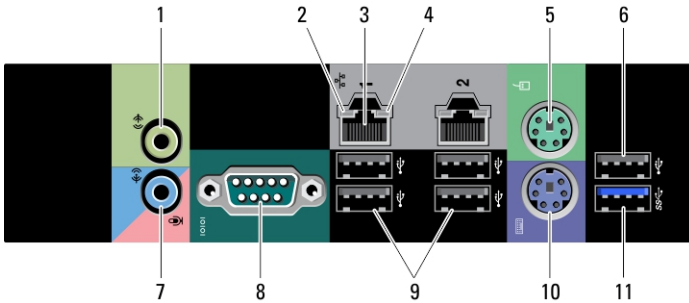
Kuva 4. Takapaneelinäkymä
